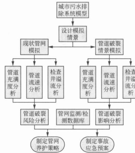
图6 管道事故分析工作流程
