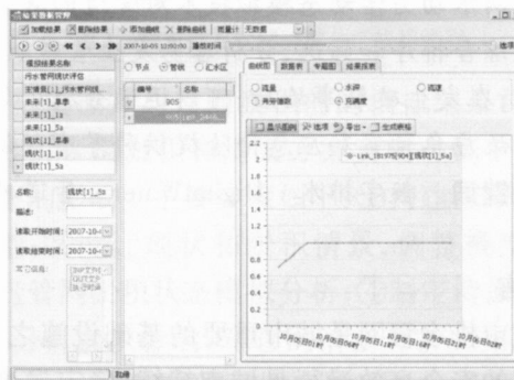
图 4 破裂管道充满度变化曲线
